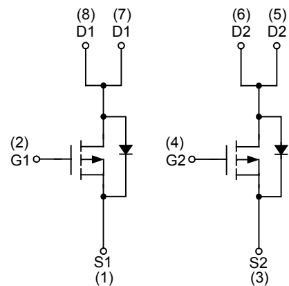
P-Channel MOSFET
