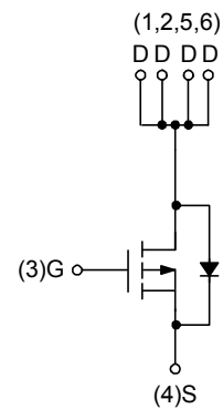
P-Channel MOSFET
