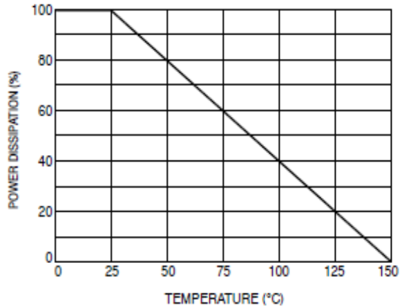
图 1 最大连续功率损耗
